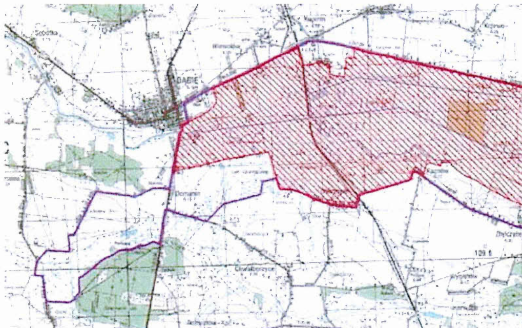
Rys.23. Pradolina Bzury - Neru Dolina na terenie Powiatu Kolskiego [źródło: RDOŚ]
