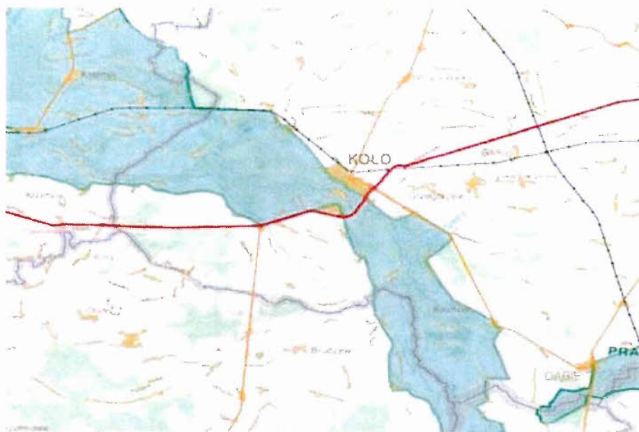
Rys.22. Dolina Środkowej Warty na terenie Powiatu Kolskiego [źródło: RDOŚ]
