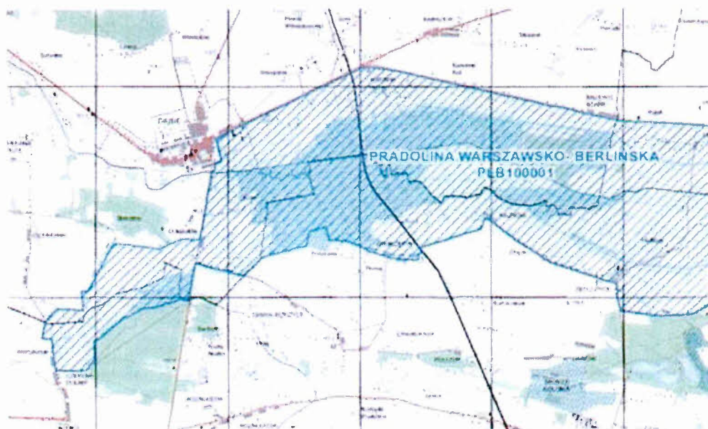
Rys.21. Pradolina Warszawsko Berlińska na terenie Powiatu Kolskiego [źródło: RDOS]
